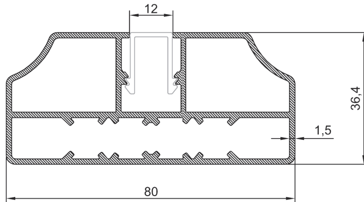
ER 5102 1,450 kg/m
