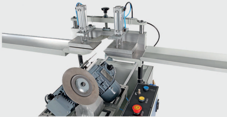
45° ALÜMİNYUM ÇITA KESME MAKİNESİ (ER-ÇKM1)
